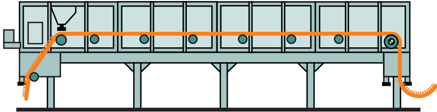
Horizontal steamer sections Horizontaldämpfer in Segmentbauweise
